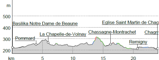
Profil altimétrique
